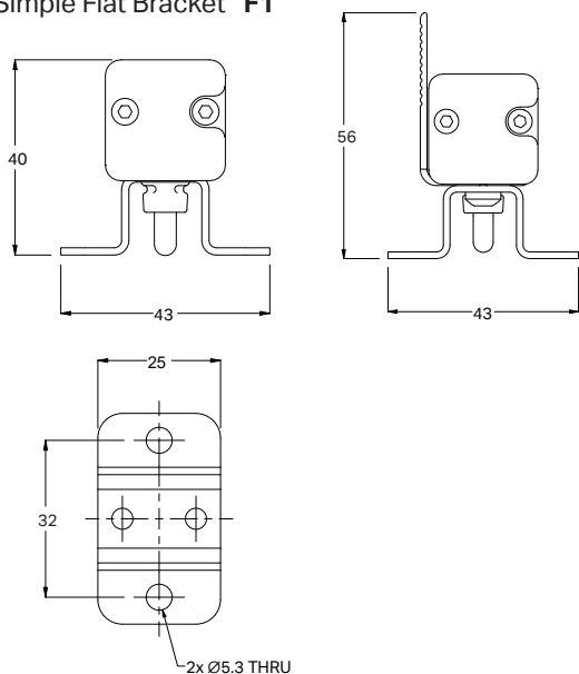
Simple Flat Bracket F1
